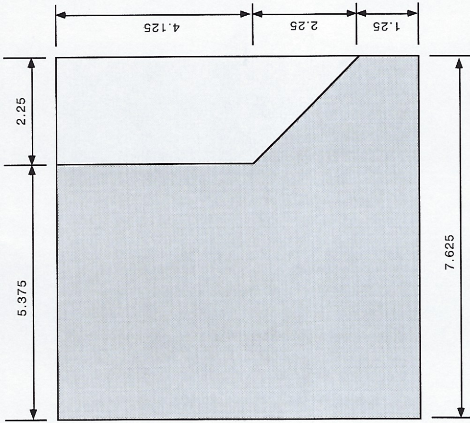
LEFT-SIDE VIEW SCALE: 1/2" = 1"
